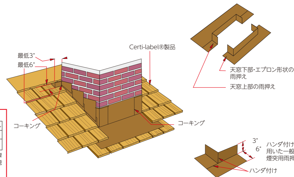
図14c : 典型的な突起物廻りの雨押え
