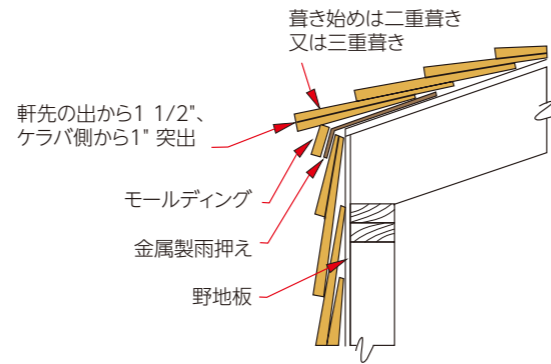
図9: 山折れ部分の接合
