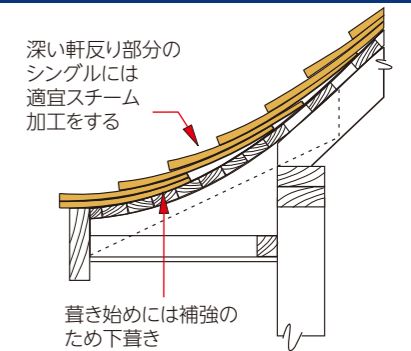
図12: 軒反り
