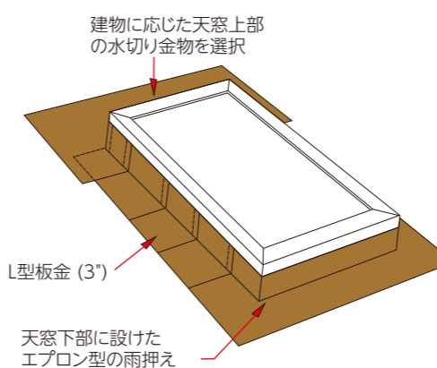
図14a : 天窗廻りの雨押え
