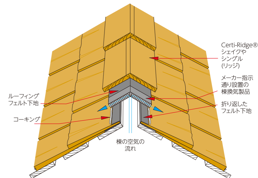
図16：棟換気
