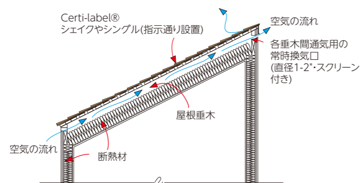
図15c：片流れ屋根
