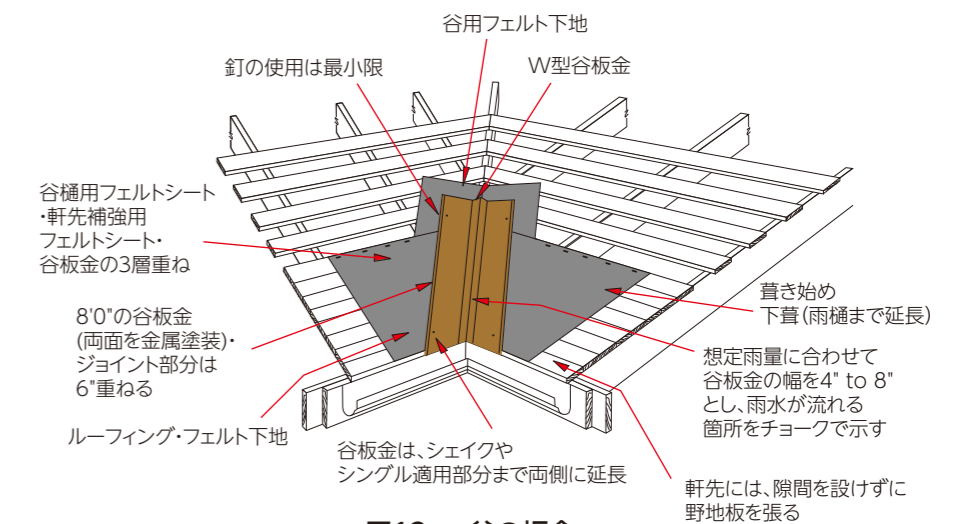
図13a: 谷の板金
