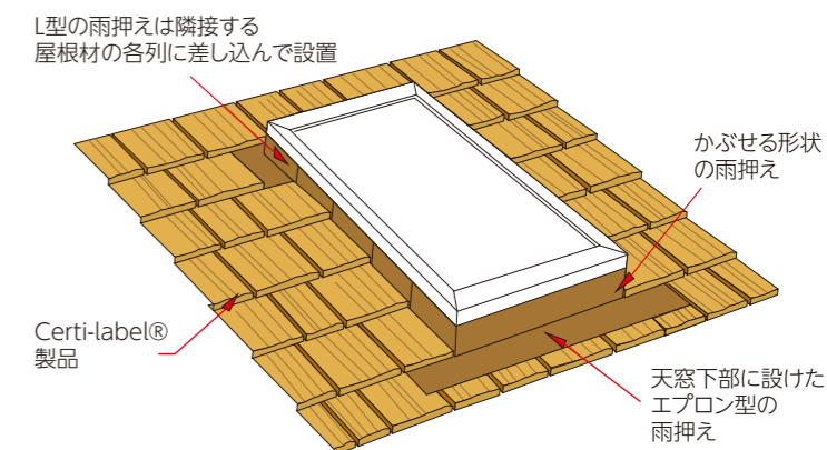
図14b : 天窗廻りの設置方法
