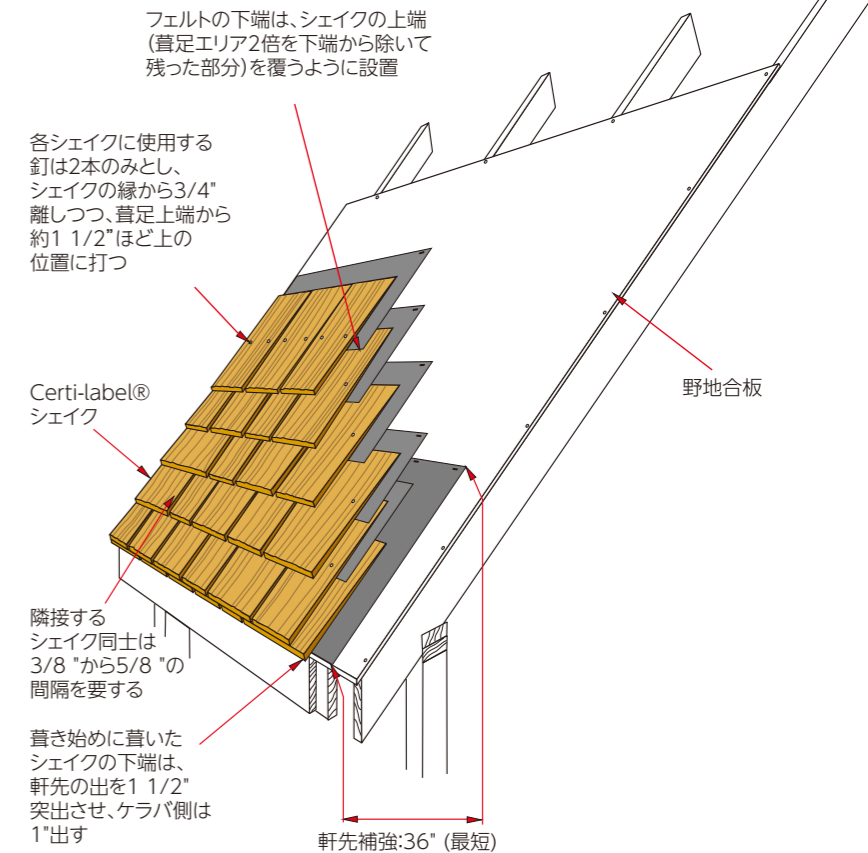
図6: マンサード屋根
